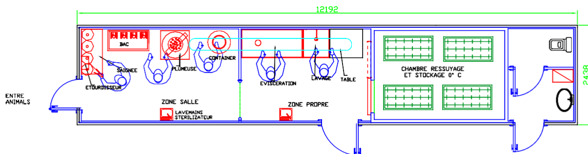
MODULE ABATTAGE VOLAILLE DE 12 METRES AVEC SERVICES
