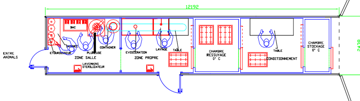
MODULE ABATTAGE VOLAILLE DE 12 METRES AVEC NR 2 CHAMBRES FROIDES
