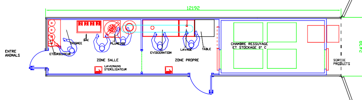
MODULE ABATTAGE VOLAILLE DE 12 METRES NR. 1 CHAMBRE FROIDE
